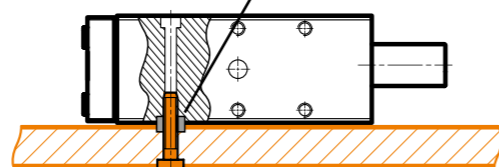
Монтаж плашмя, с помощью винтов снизу
